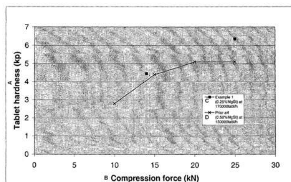
A DURETÉ DES COMPRIMÉS (KP) C EXEMPLE 1 (0,25 %MGST) À 170000TABL/H B FORCE DE COMPRESSION (KN) D ETAT DE LA TECHNIQUE (0,50 %MGST) À 150000TABL/H
