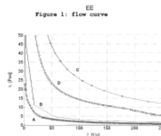
Curve A: Oil in water emulsion AA Curve B: Jellified emulsion BB Curve C: Monophase gel CC Curve D: Monophase gel DD AA Courbe A: Emulsion huile dans l'eau BB Courbe B: Emulsion gélifiée CC Courbe C: Gel monophase DD Courbe D: Gel monophase EE courbe d'écoulement
